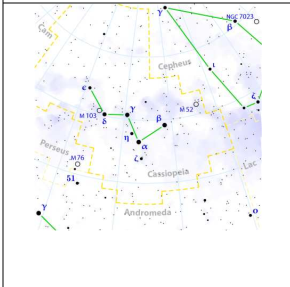
Casiopea (Cassiopeia)
