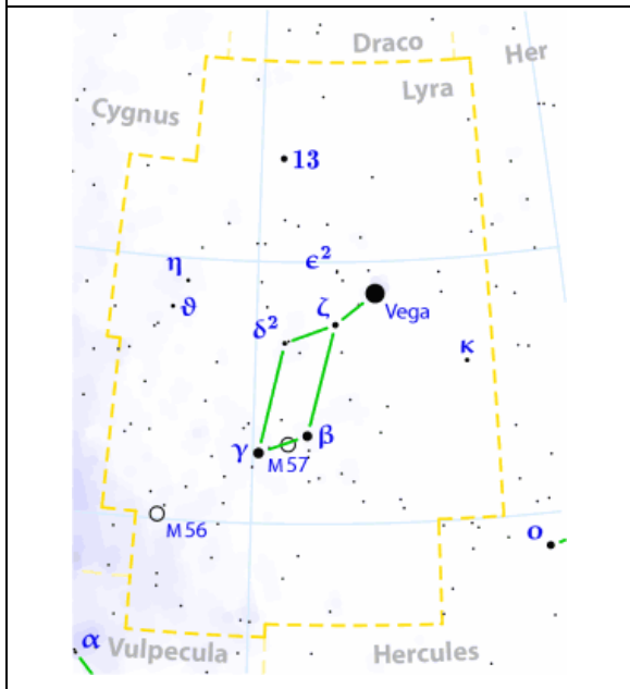
Lira (Lyra)
