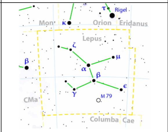
Liebre (Lepus)
