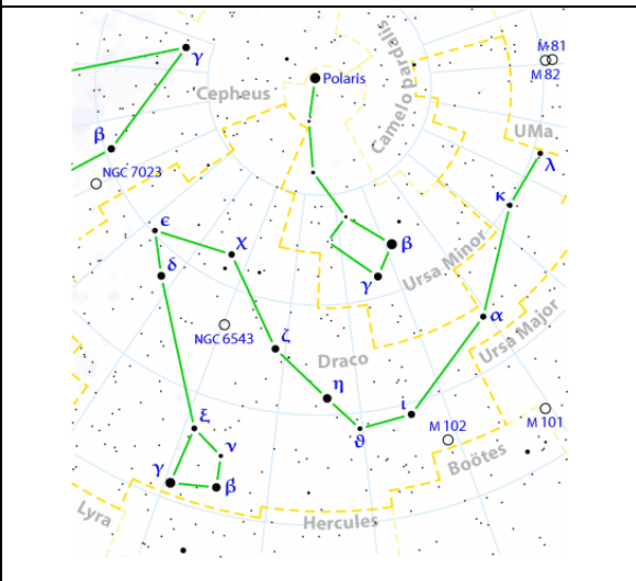
Dragón (Draco)
