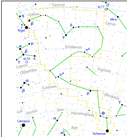
Eridano (Eridanus)
