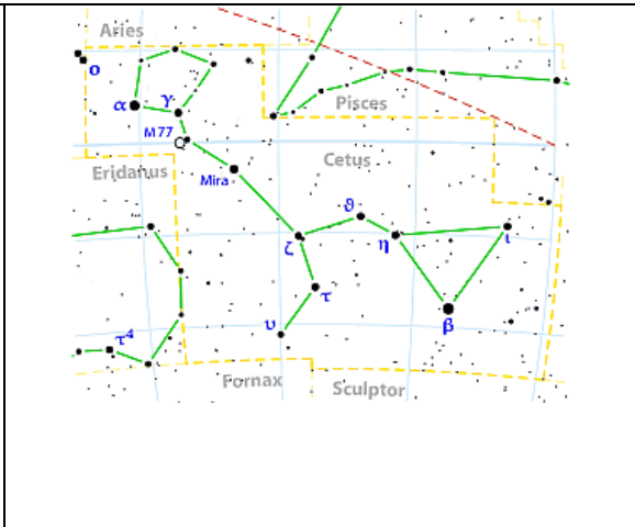
Ballena (Cetus)
