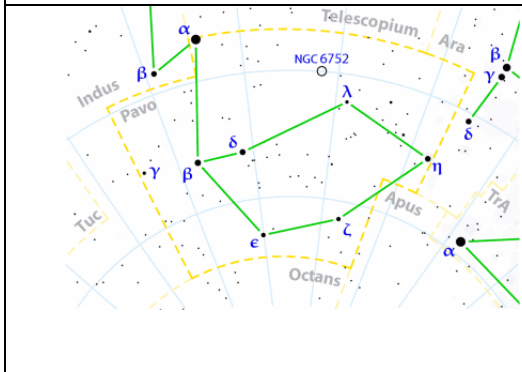
Pavo (Pavo)
