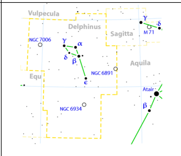
Delfín (Delphinus)
