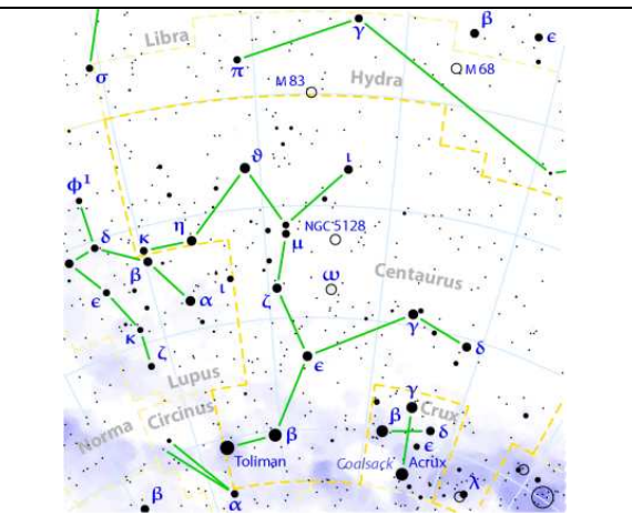
Centauro (Centaurus)
