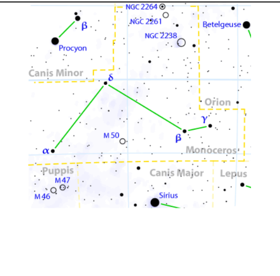
Unicornio (Monoceros)
