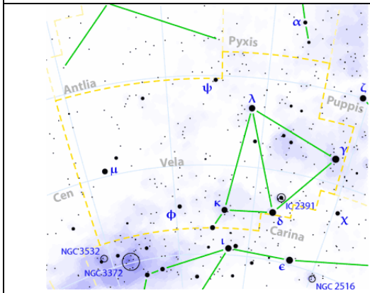
Vela (Vela)
