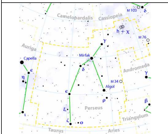
Perseo (Perseus)
