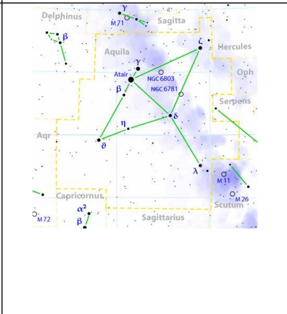
Águila (Aquila)
