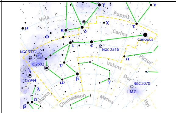
Quilla (Carina)
