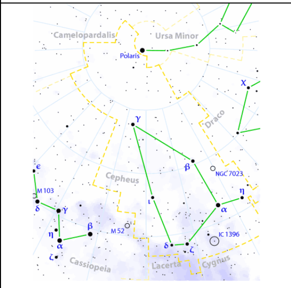
Cefeo (Cepheus)
