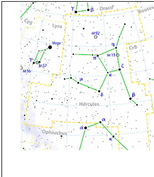
Hércules (Hercules)
