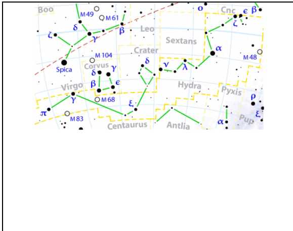
Hidra (Hydra)
