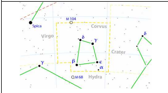
Cuervo (Corvus)
