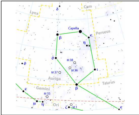
Cochero (Auriga)
