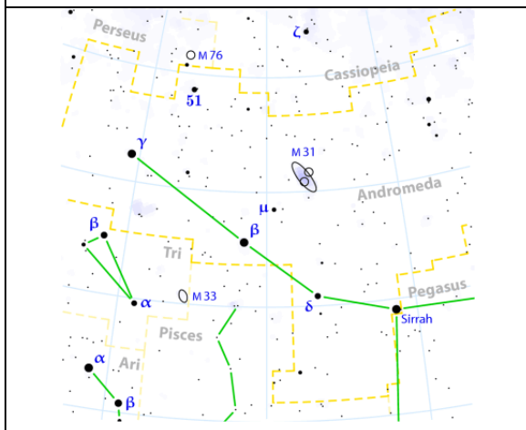
Andr6meda (Andromeda)
