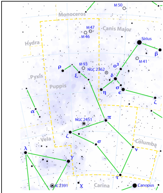
Popa (Puppis)
