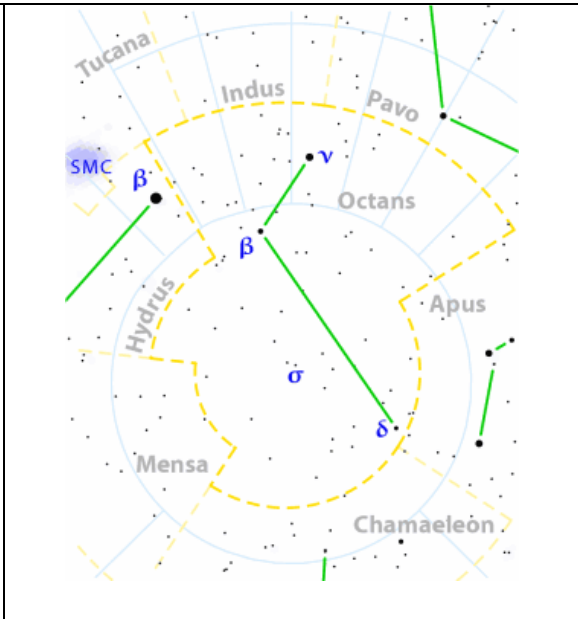
Octante (Octans)
